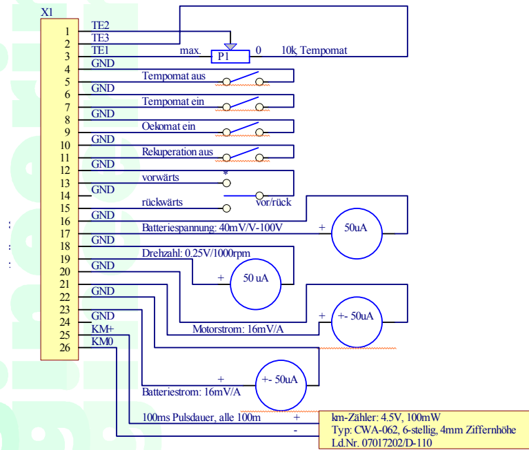
Variante 1 mit nur einem Pedal
