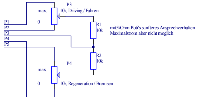
Variante 2 mit separatem Bremspedal
